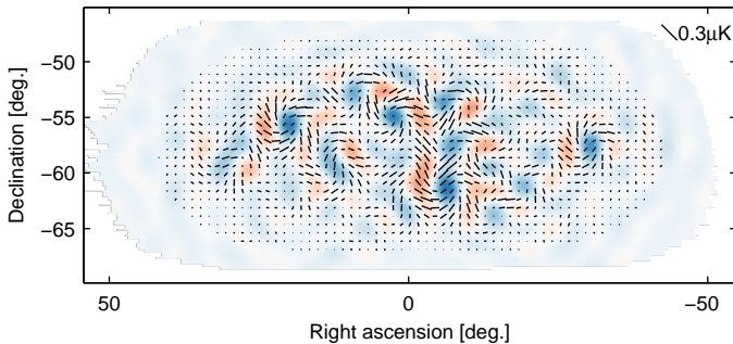
Keck Array : B signal
