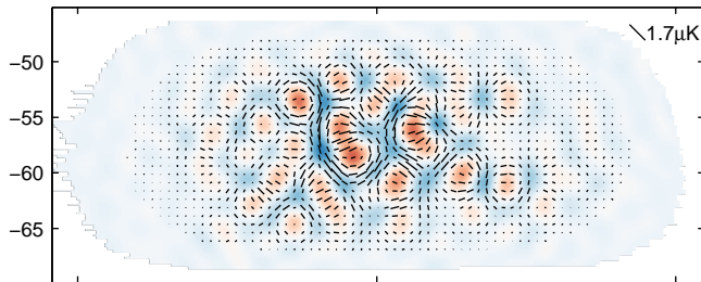
Keck Array : B signal
