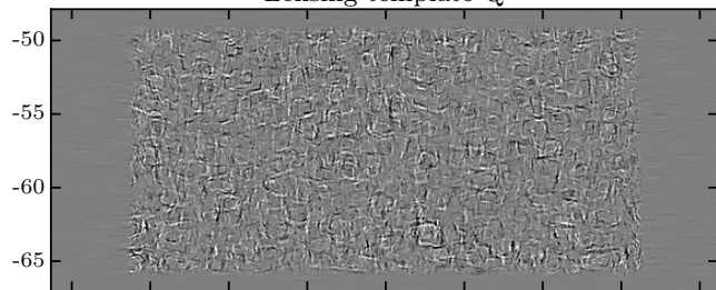
Lensing template Q
