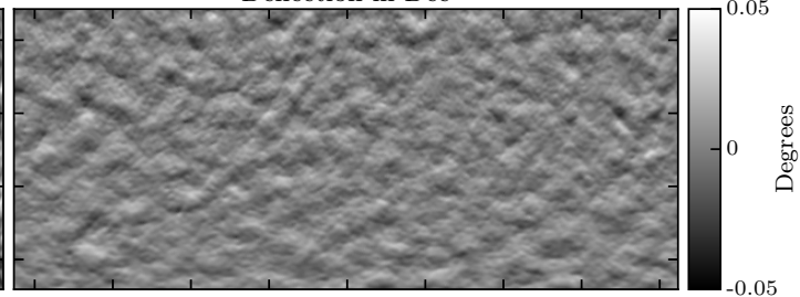
Lensing template U
