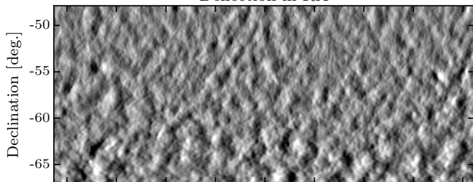
Lensing template Q
