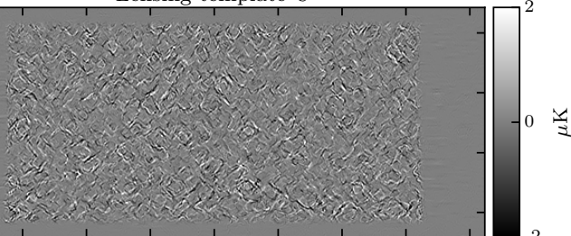
Lensing template U
