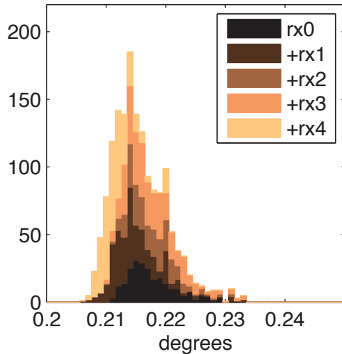
Keck 2013 Beam Width
