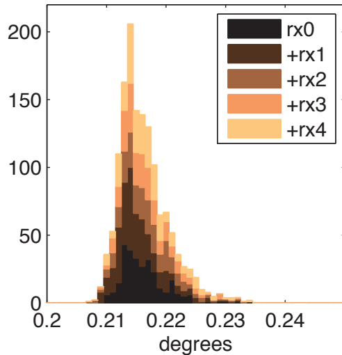
Keck 2012 Beam Width
