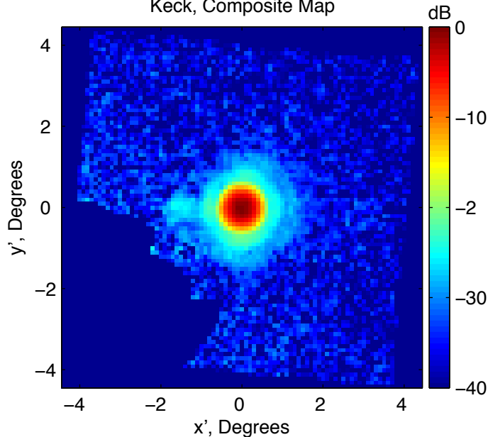
Keck, Composite Map
