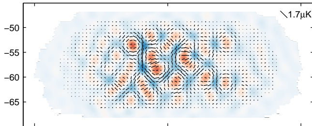
BICEP2: B signal
