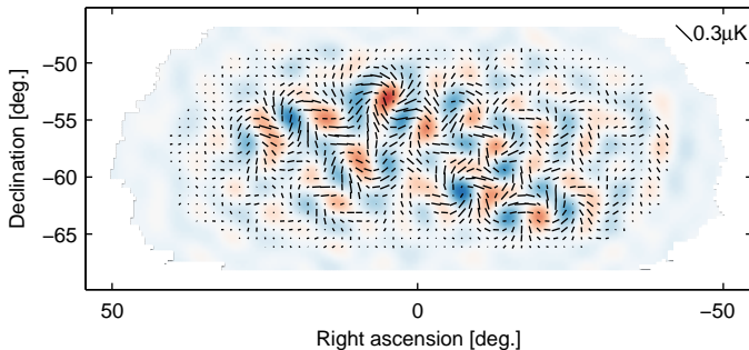
BICEP2: B signal
